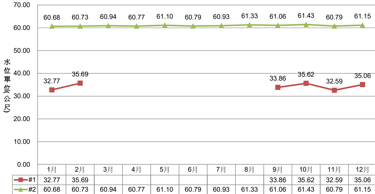
金酒公司金寧廠111年地下水井#1、#2水位監測年報圖表
